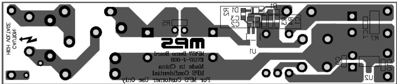
Figure 3—Bottom Layer
