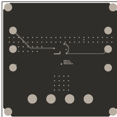
Figure 4—Bottom Layer
