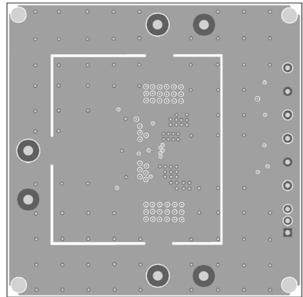
Inner1 Layer
