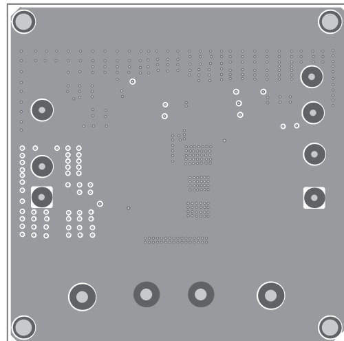
Figure 4—IN2 Layer
