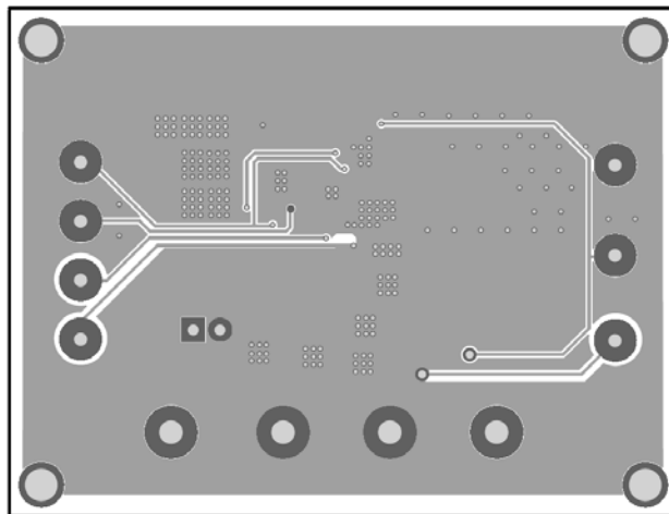
Figure 3—Bottom Layer
