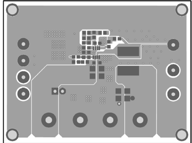
Figure 2—Top Layer
