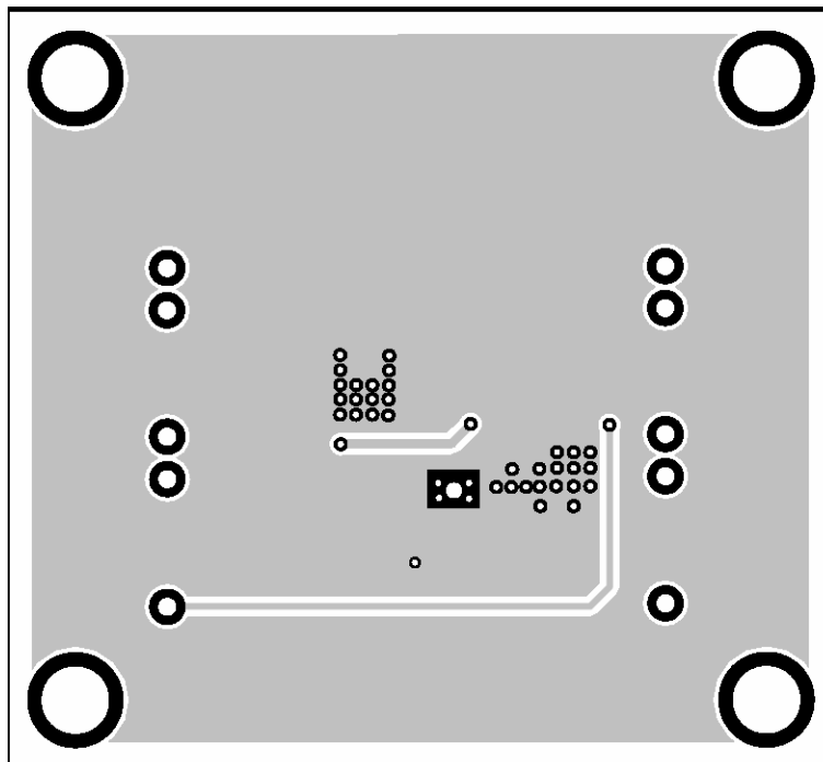
Figure 2—Bottom Layer
