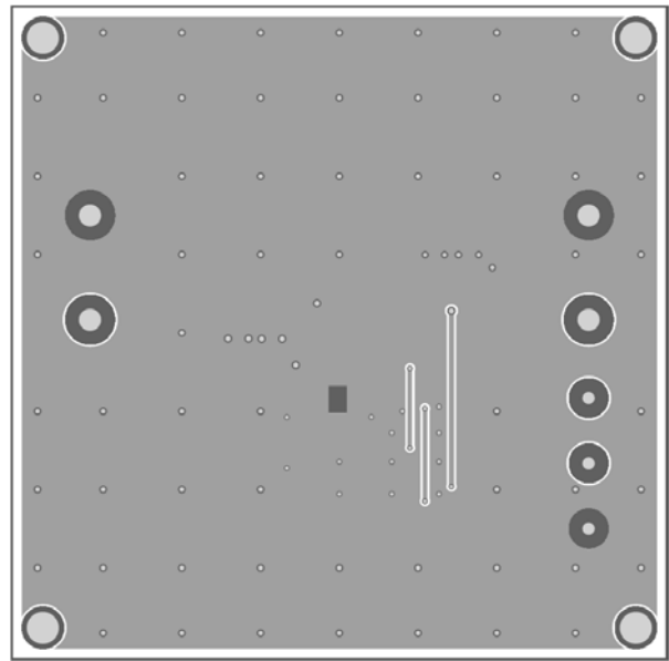
Figure3 – Bottom Layer
