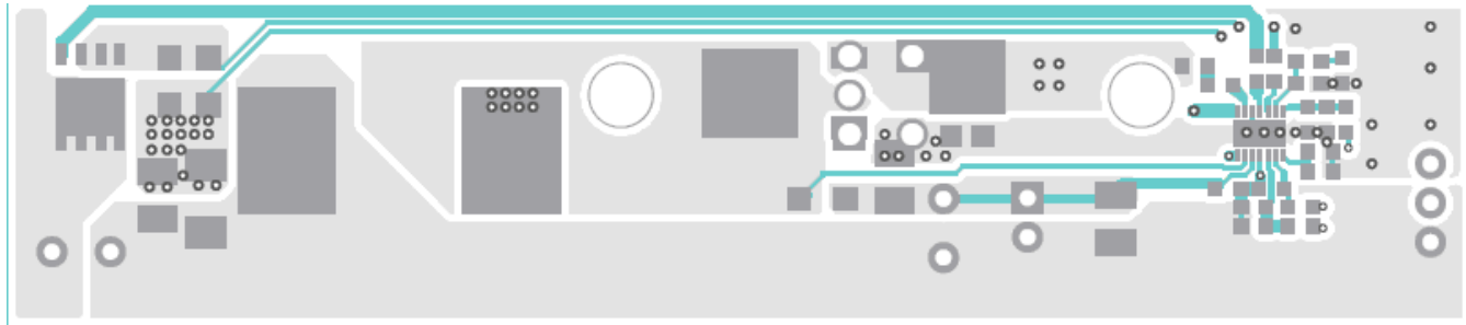
Figure 3—Top Layer
