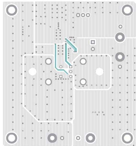
Figure 4—Bottom Layer
