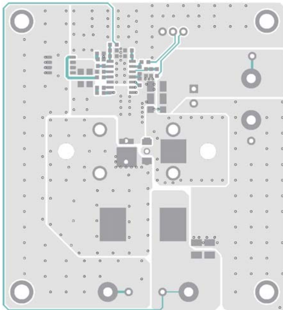
Figure 3—Top Layer
