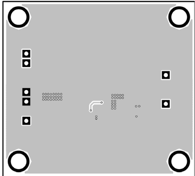
Figure 2—Bottom Layer
