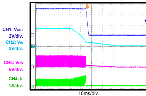
VIN Shutdown
