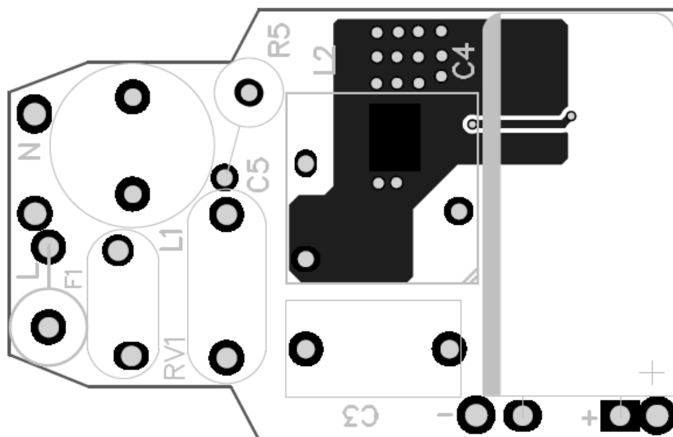
Figure 2—Top Layer
