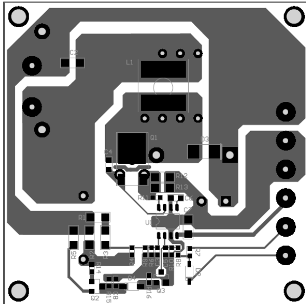
Figure 4—Bottom Layer
