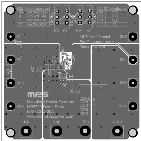
Figure 1—Top Layer
