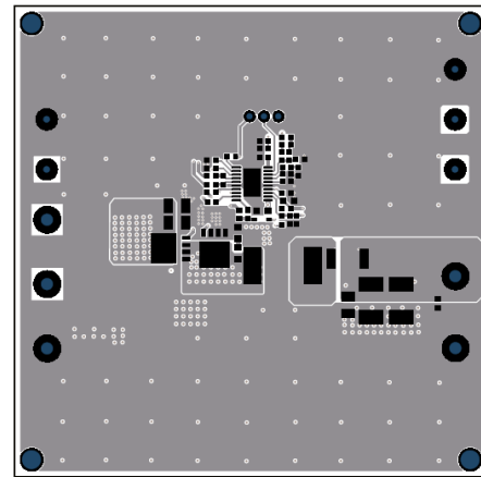
Figure 2—Top Layer
