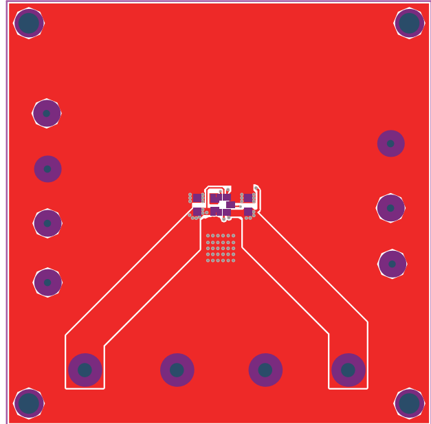
Figure 4—Top Layer
