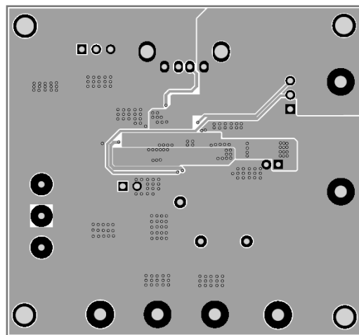
Figure 5—Bottom Layer
