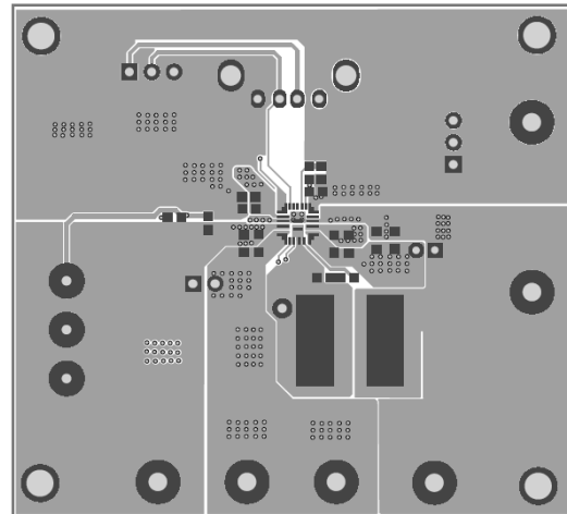
Figure 2—Top Layer
