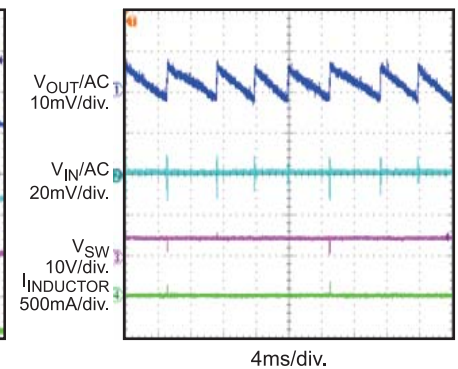
Input / Output Ripple
