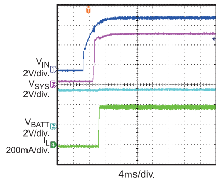
En Off, Charge Mode
