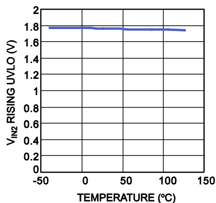
V_{IN2} Rising UVLO
