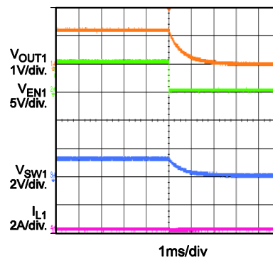
EN Down without Load (CH1)
