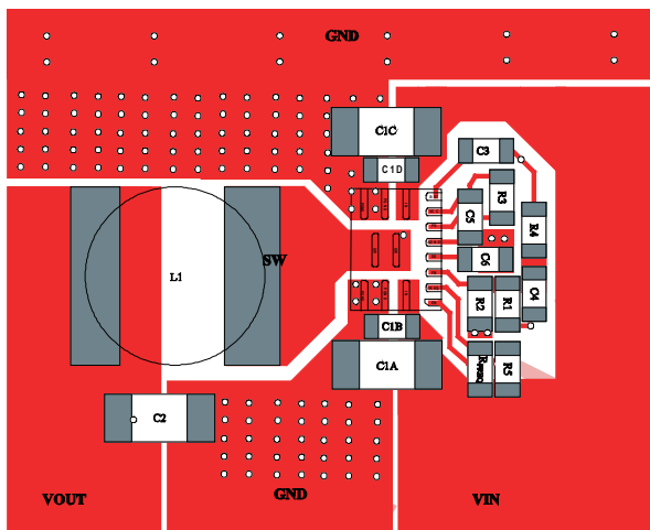
Top Layer
