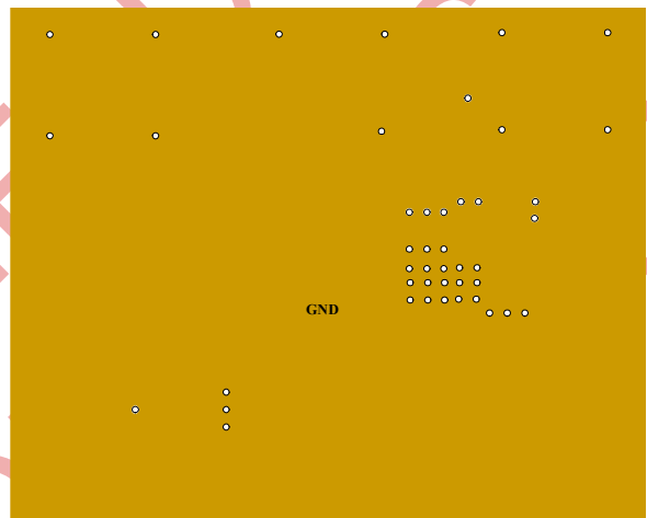
Inner1 Layer
