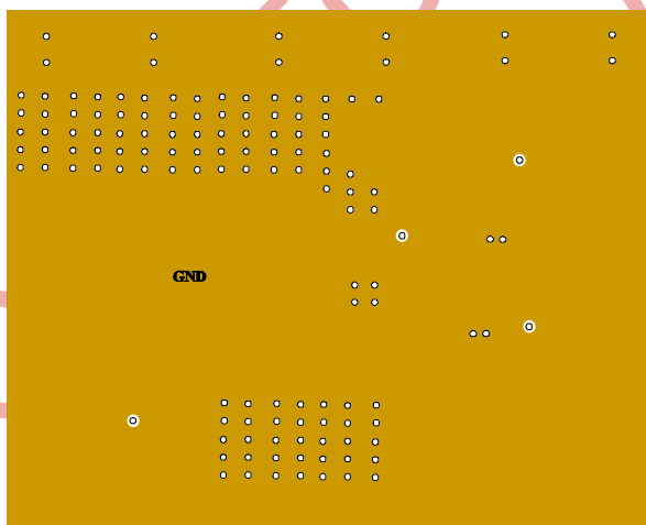
Inner1 Layer
