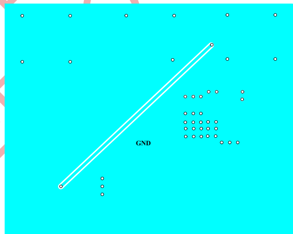
Inner2 Layer
