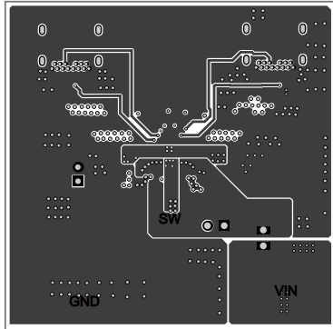
Middle Layer 1
