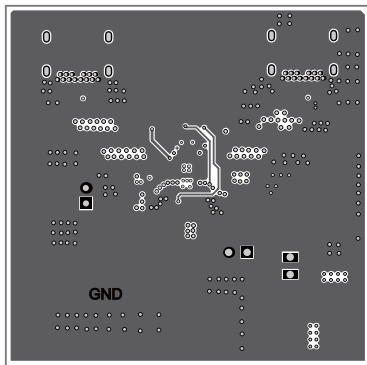
Middle Layer 2
