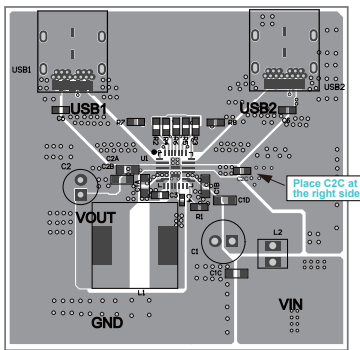
Top Layer
