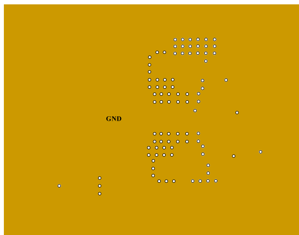
Inner1 Layer
