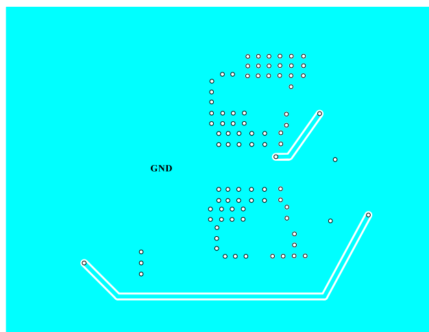
Inner2 Layer
