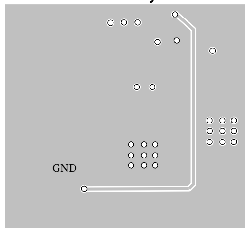
Inner2 Layer
