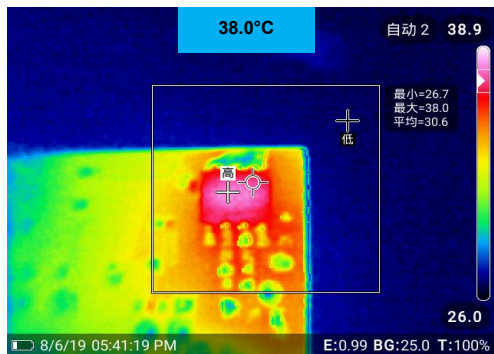
Thermal V_{IN}=85V_{AC}
