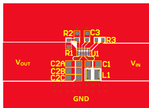
Top Layer
