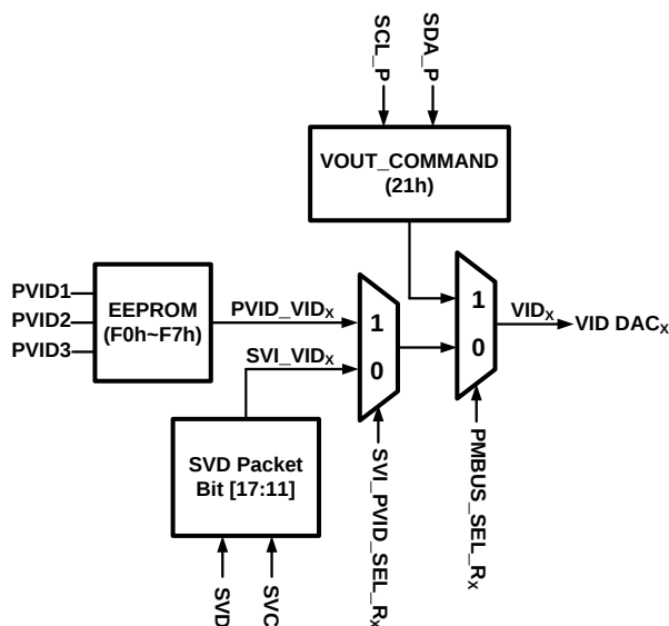
Figure 4: VID Control
