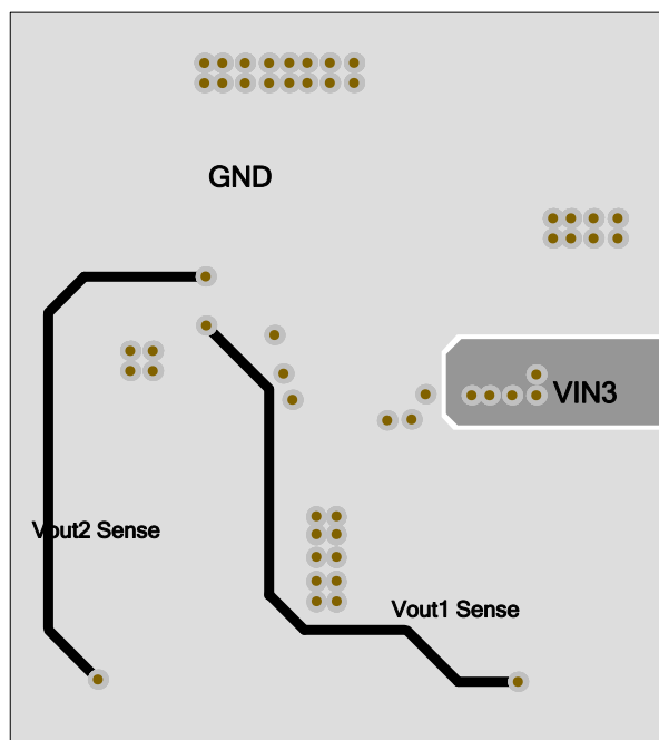
Bottom Layer
