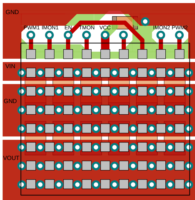
Top Layer
