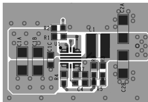
Top Layer
