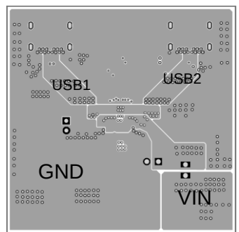
Bottom Layer
